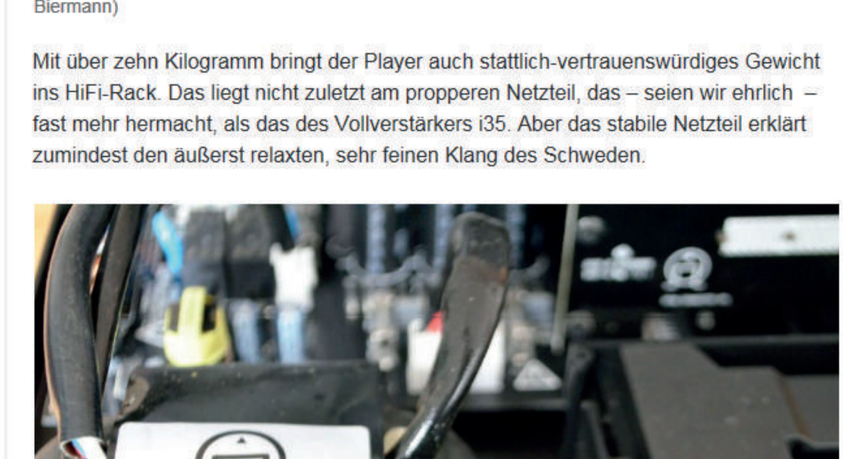
Erstaunlich kräftig: der Trafo des CD35 ist größer als der des Vollverstärkers i35 und sorgt für jederzeit ausreichende Spannungsverhältnisse (Foto: H. Biermann)
